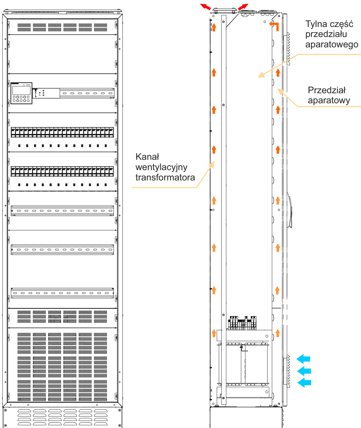
Cyrkulacyjny sposób chłodzenia transformatora
